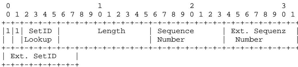
Figure 10: TinyIPFIX Message Header Format if E1 = E2 = 1
